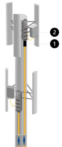
FTTA-Anschlusskästen und Jumper für RRU-Anschluss.
