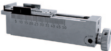
Aufnahme für Fujikura Faserhalter
