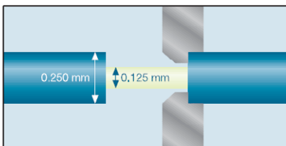
Die Faser wird abisoliert, ohne dass das Messer das Glas berührt.
