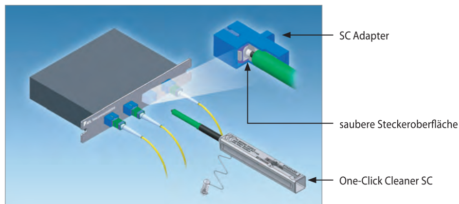
Illustration des Reinigungsvorgangs am Beispiel eines SC Steckers
