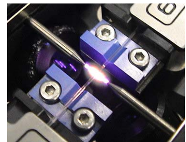
Spleiss zweier 400µm Fasern
